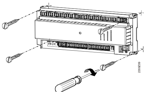
Přišroubování
