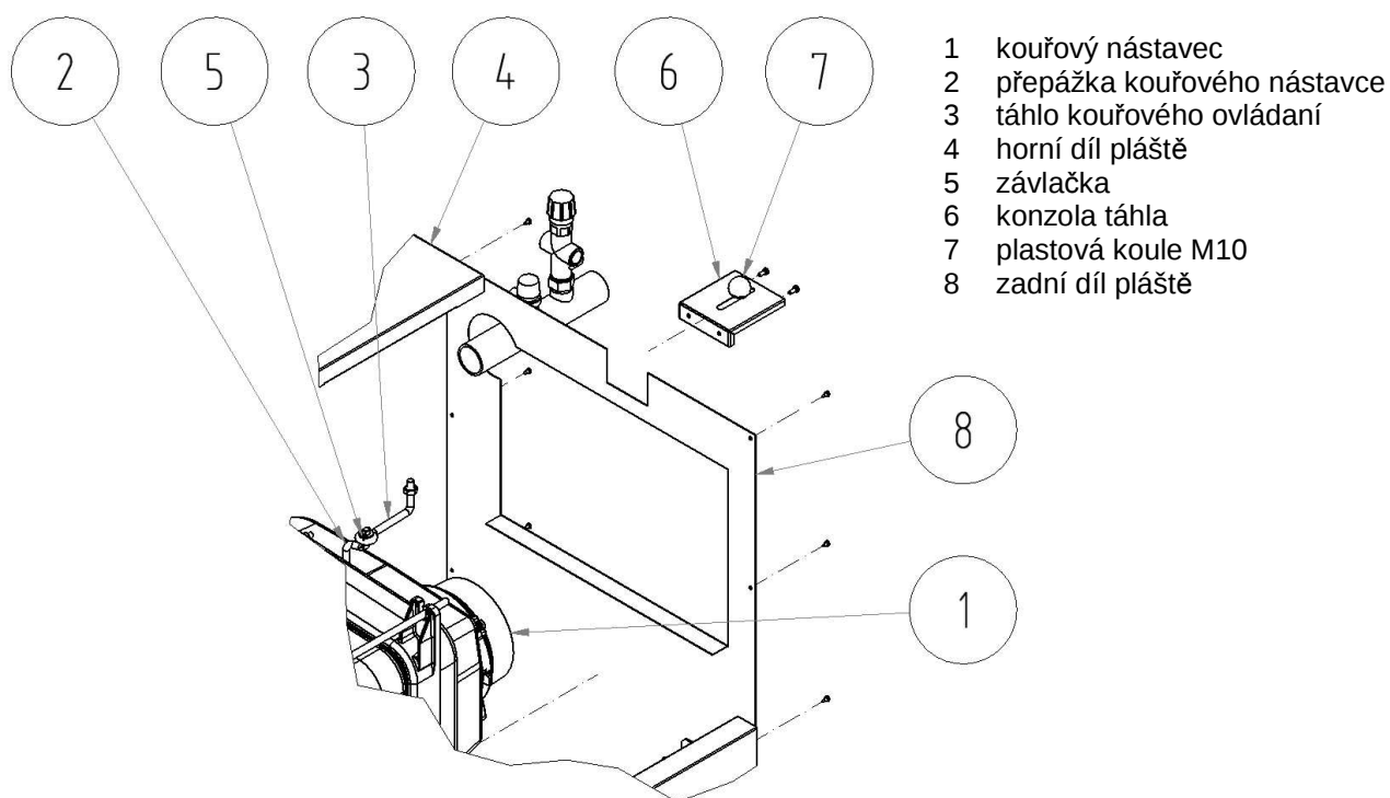
Obr. č. 8 Montáž ovládaní táhla kouřového ovládaní
