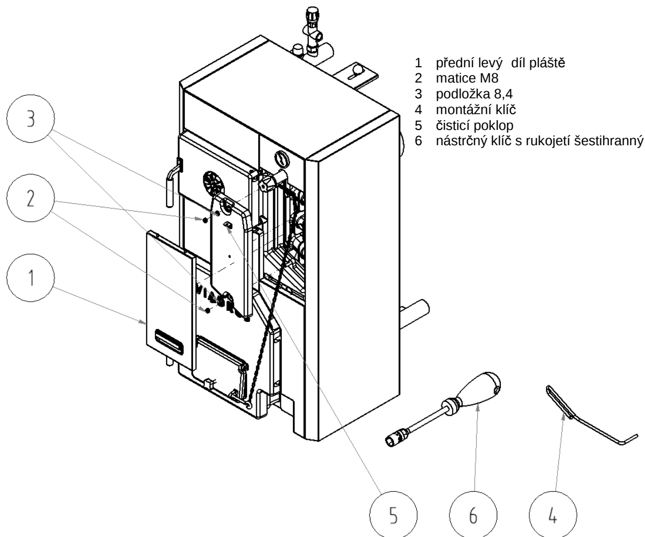
Obr. č. 13 Demontáž čisticího poklopu
